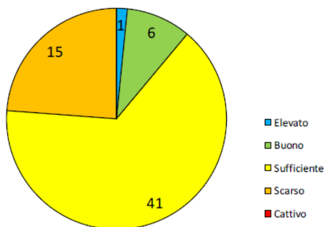
Immagine n. 11 (Estratta da Rapporto tecnico acque superficiali – 2013 - ARPAV)
