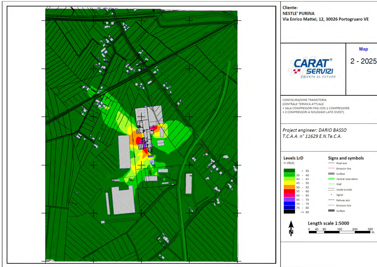
Figura 27 MAPPA IN PIANTA IMPATTO ACUSTICO STATO TRANSITORIO (SORGENTI FISSE: CENTRALE TERMICA + SALA COMPRESSORI PKG + 2 COMPRESSORI A NOLEGGIO) – PERIODO DIURNO/NOTTURNO
