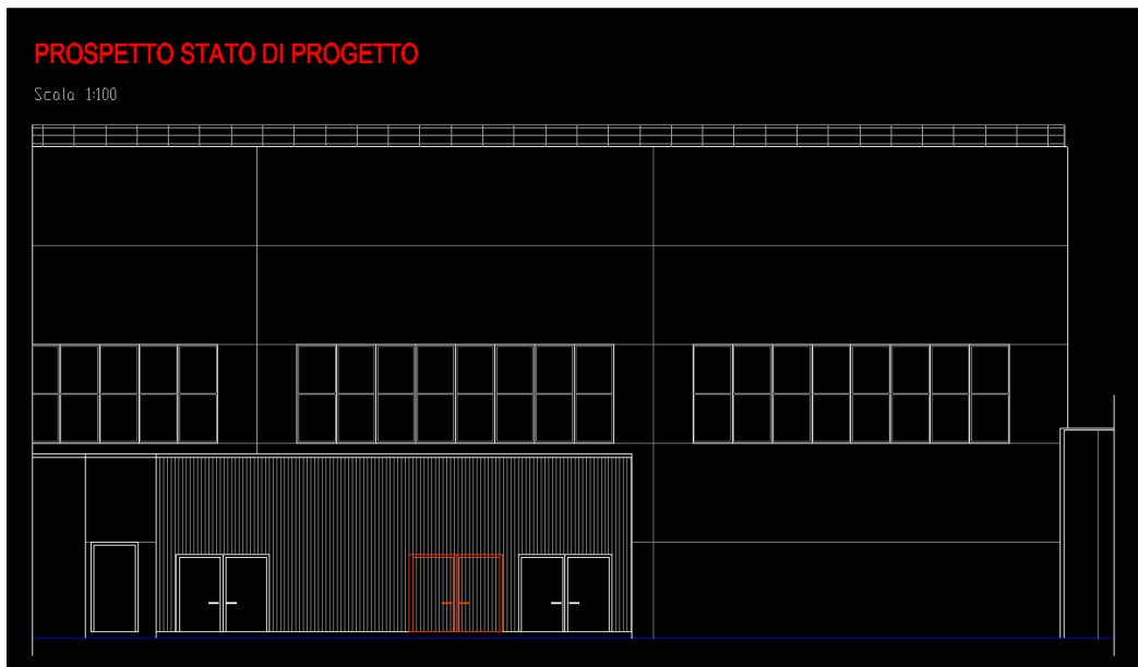
Figura 40 Sala compressori PKG – prospetto stato di progetto
