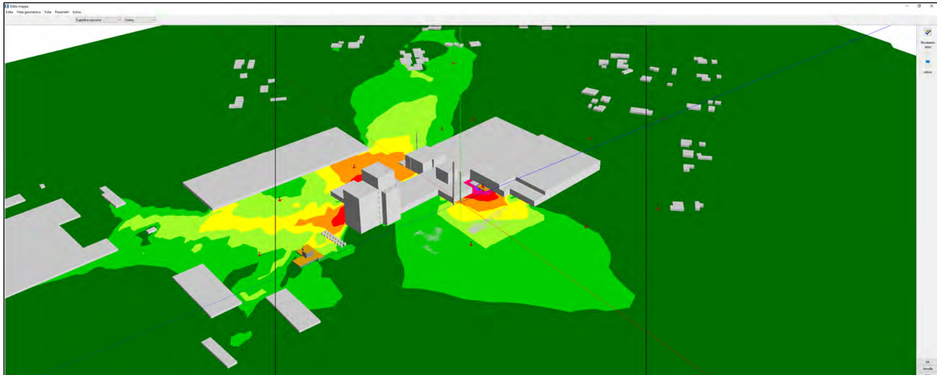
Figura 29 MAPPA 3D IMPATTO ACUSTICO STATO TRANSITORIO (SORGENTI FISSE: CENTRALE TERMICA + SALA COMPRESSORI PKG + 2 COMPRESSORI A NOLEGGIO) – PERIODO DIURNO/NOTTRUNO – LATO EST
