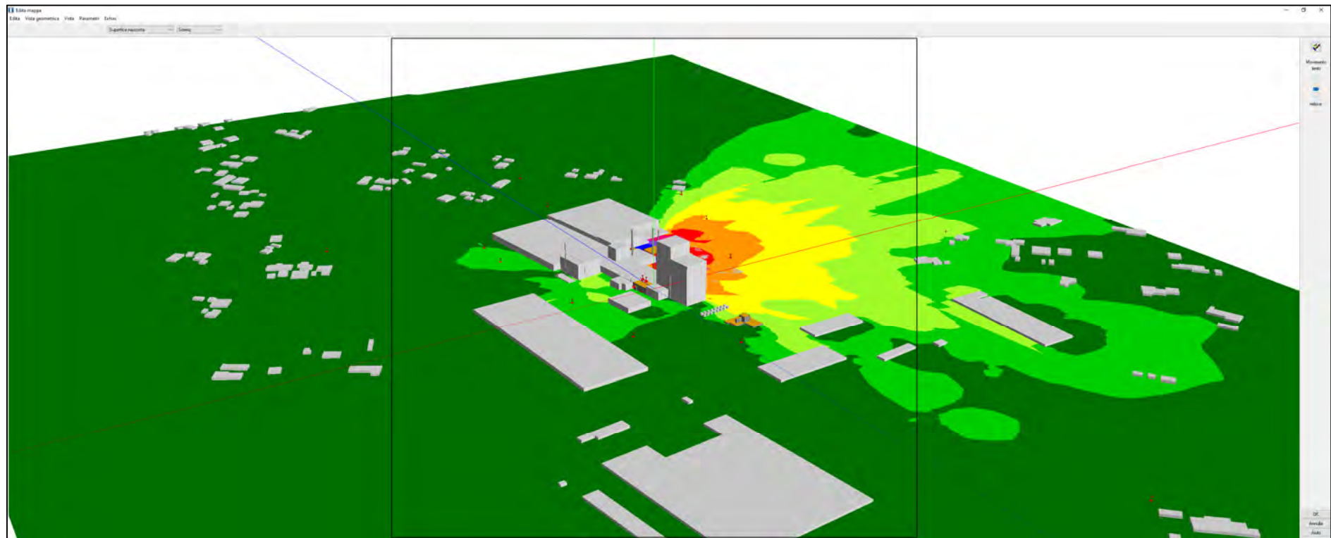
Figura 46 MAPPA 3D IMPATTO ACUSTICO STATO DI PROGETTO (SORGENTI FISSE: NUOVA CENTRALE TERMICA + SALA COMPRESSORI PKG CON 4 COMPRESSORI E 4 ESTRATTORI D'ARIA) – PERIODO DIURNO / NOTTURNO – LATO OVEST
