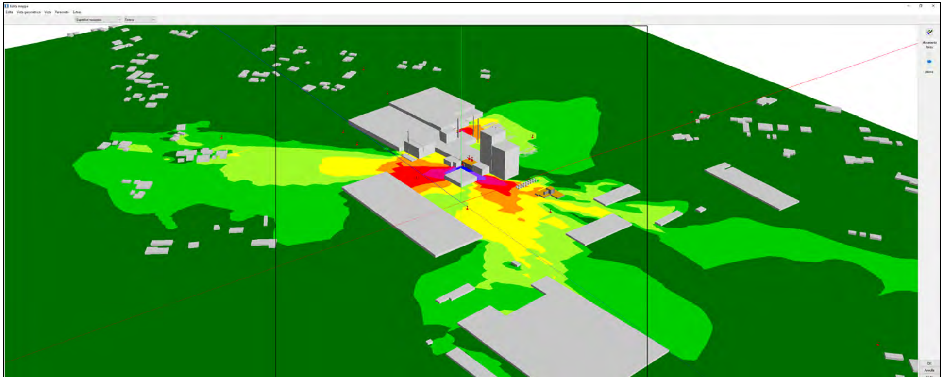
Figura 17 MAPPA 3D IMPATTO ACUSTICO STATO DI FATTO 2025 (SORGENTI FISSE: CENTRALE TERMICA + SALE COMPRESSORI KAESER E PKG) – PERIODO DIURNO/NOTTRUNO – LATO OVEST
