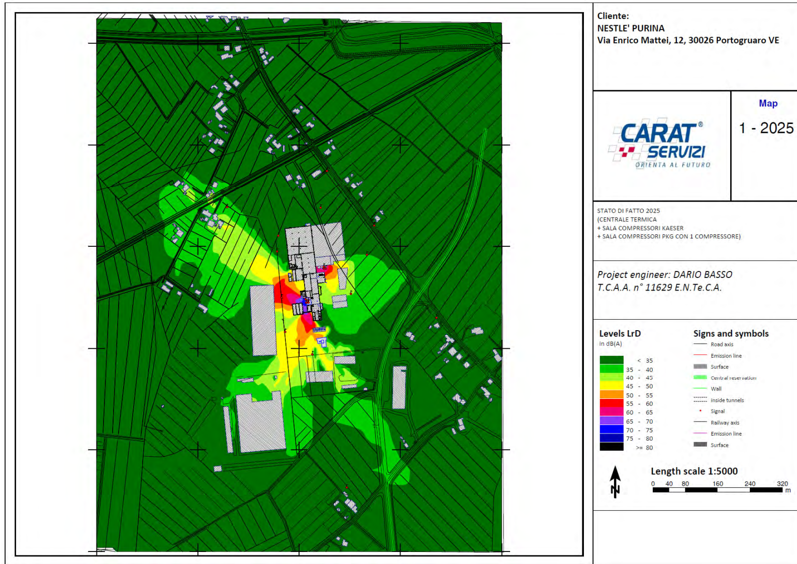
Figura 16 MAPPA IN PIANTA IMPATTO ACUSTICO STATO DI FATTO 2025 (SORGENTI FISSE: CENTRALE TERMICA + SALE COMPRESSORI KAESER E PKG) – PERIODO DIURNO/NOTTRUNO
