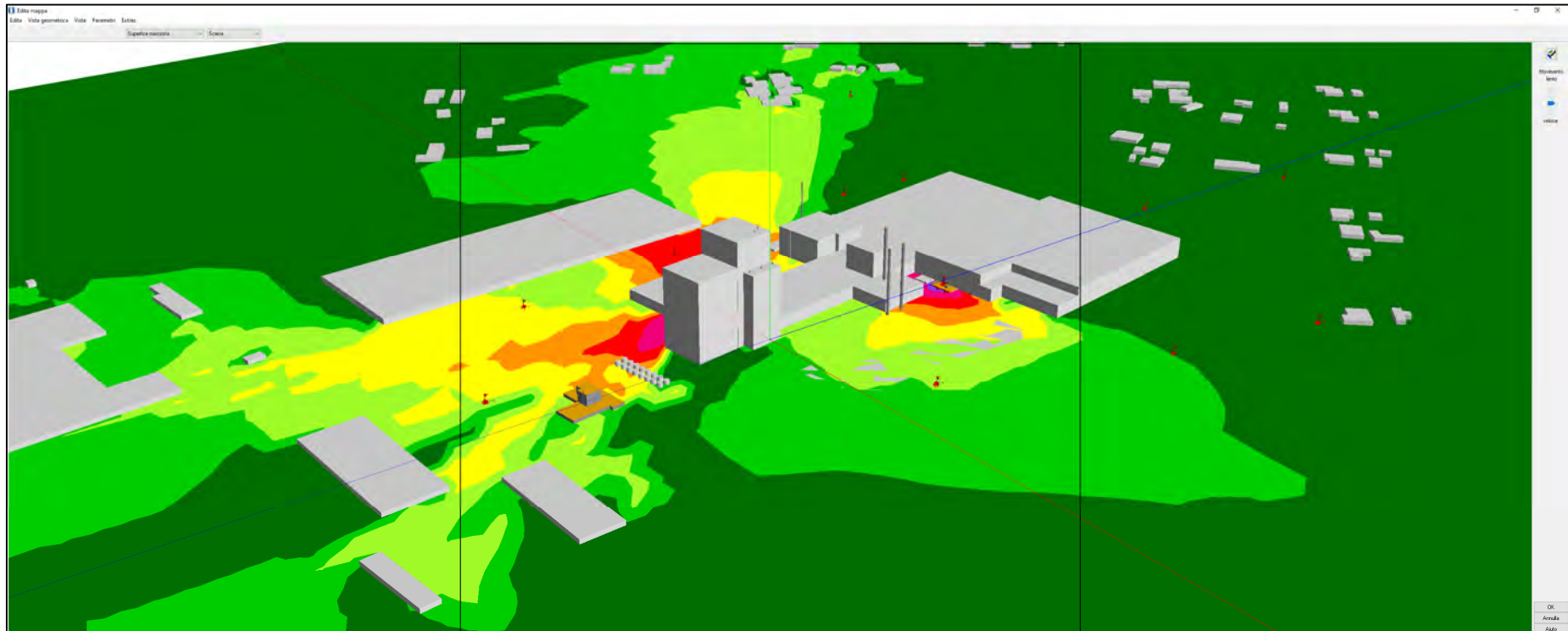
Figura 18 MAPPA 3D IMPATTO ACUSTICO STATO DI FATTO 2025 (SORGENTI FISSE: CENTRALE TERMICA + SALE COMPRESSORI KAESER E PKG) – PERIODO DIURNO/NOTTRUNO – LATO EST
