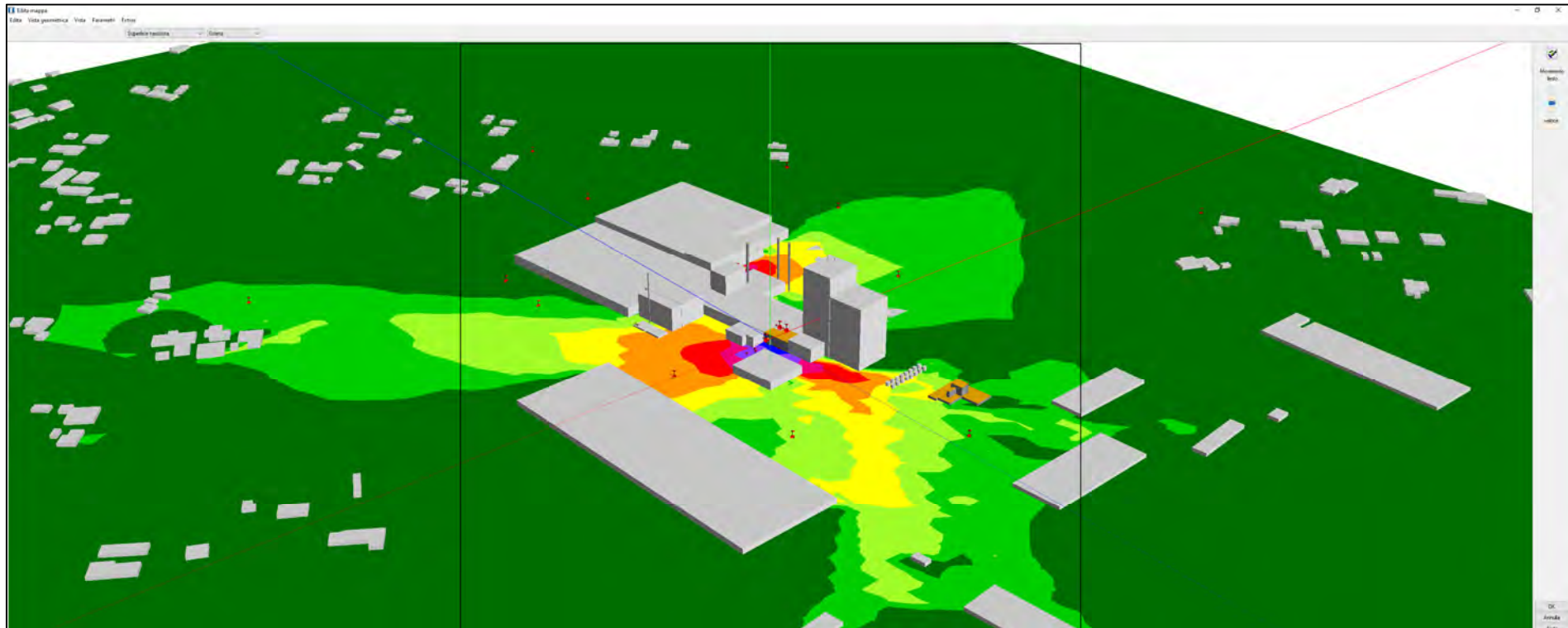
Figura 28 MAPPA 3D IMPATTO ACUSTICO STATO TRANSITORIO (SORGENTI FISSE: CENTRALE TERMICA + SALA COMPRESSORI PKG + 2 COMPRESSORI A NOLEGGIO) – PERIODO DIURNO/NOTTRUNO – LATO OVEST
