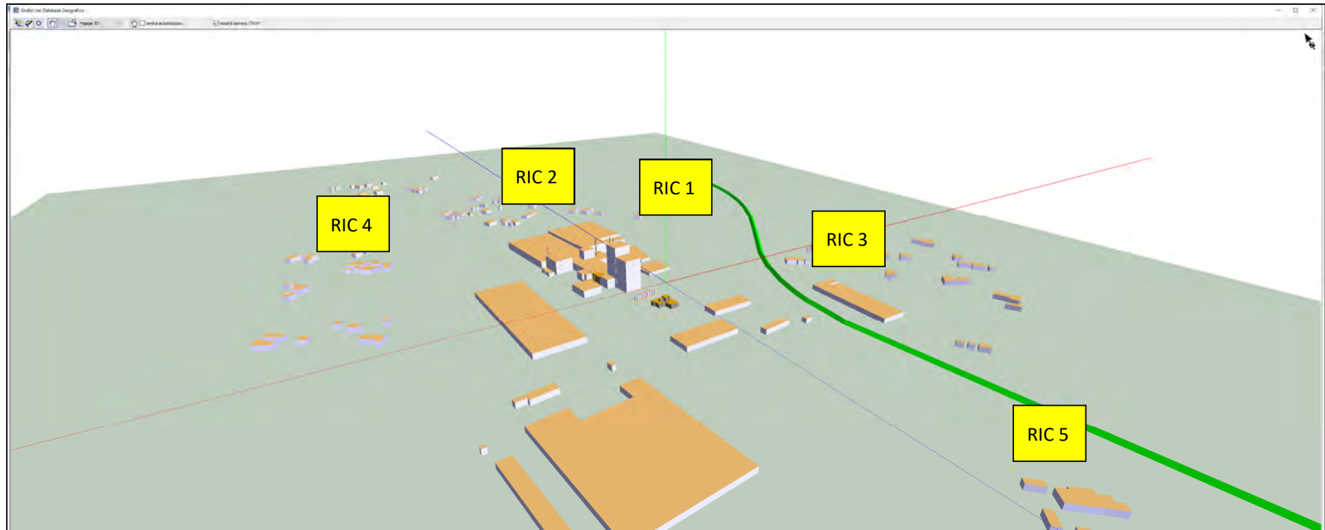
Figura 9 Vista 3D data base cartografico – con punti di verifica ai ricettori.
