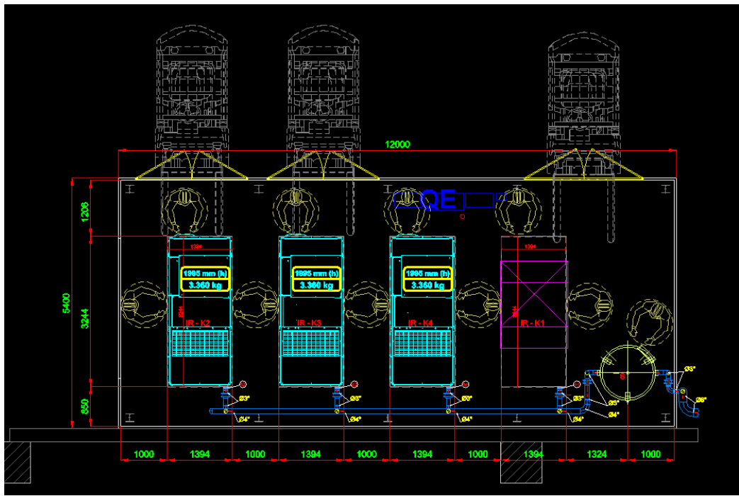
Figura 41 Sala compressori PKG – pianta stato di progetto con dettaglio posizionamento compressori
