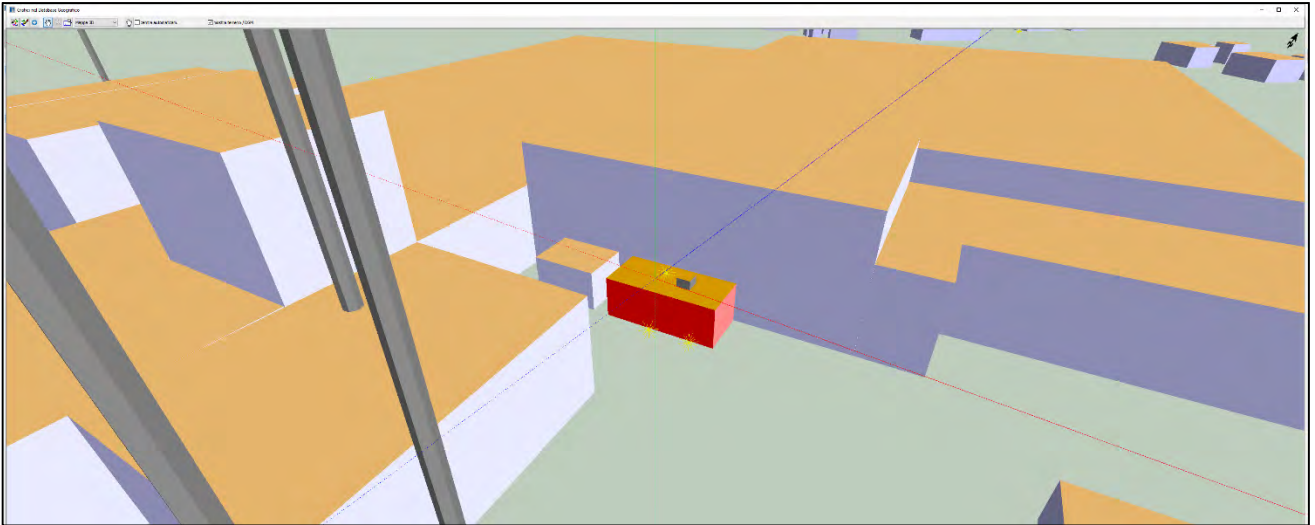
Figura 7 Vista generale sorgenti sala compressori PKG (sorgenti fisse).
