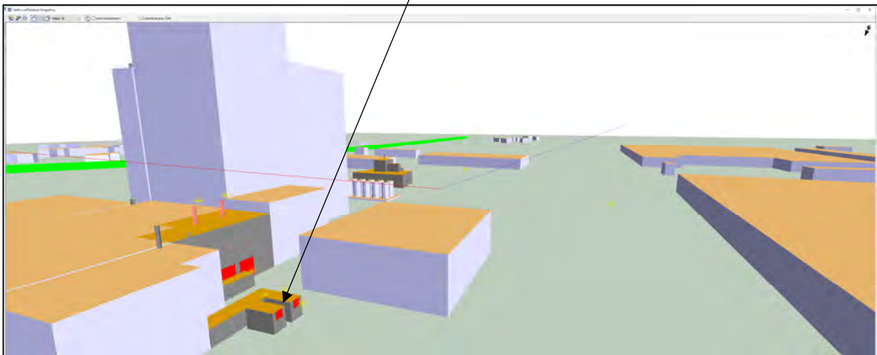
Figura 26 Mappa 3D posizionamento compressori
