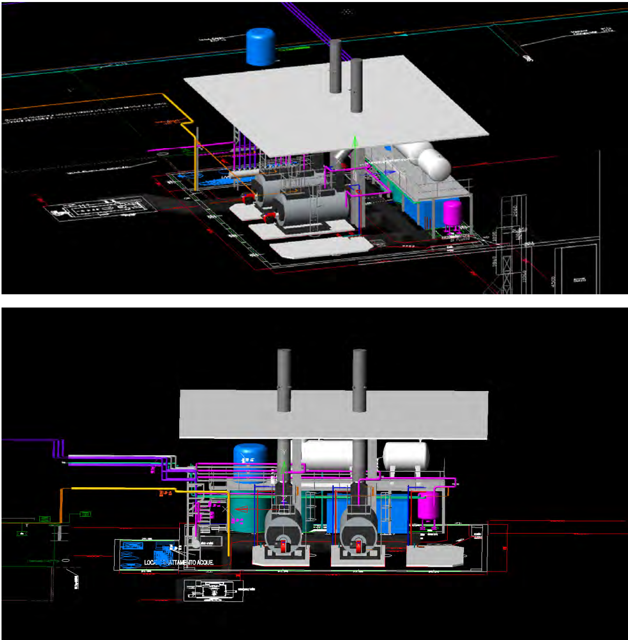
Figura 38 Nuova centrale termica - Viste 3D del progetto
