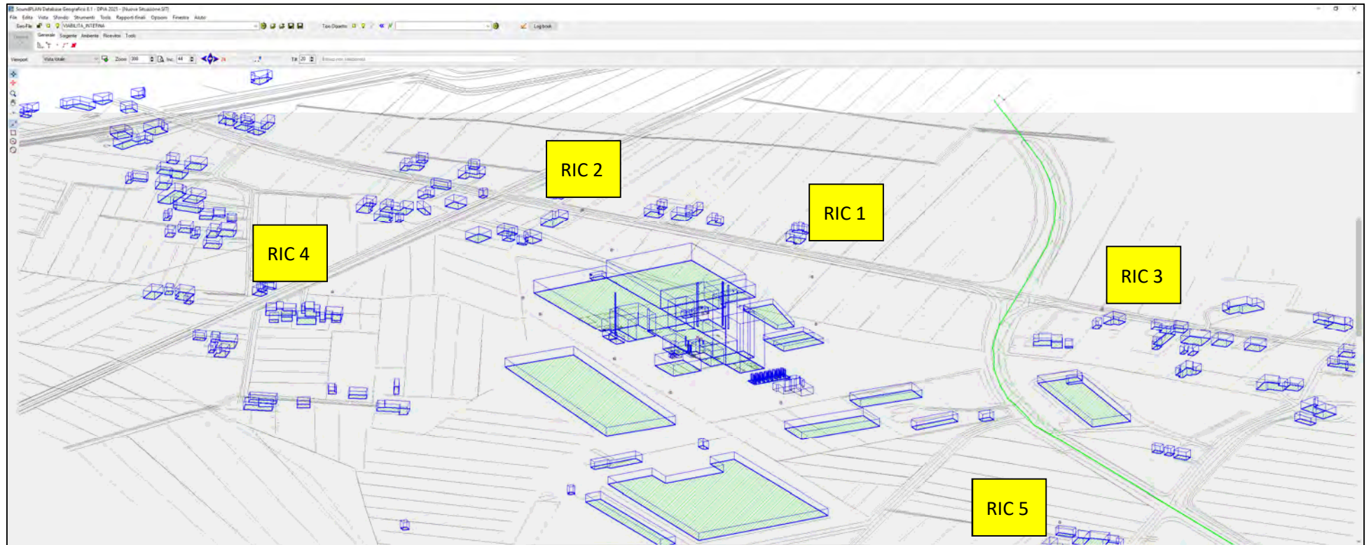
Figura 10 Vista 3D con punti di verifica ai ricettori.
