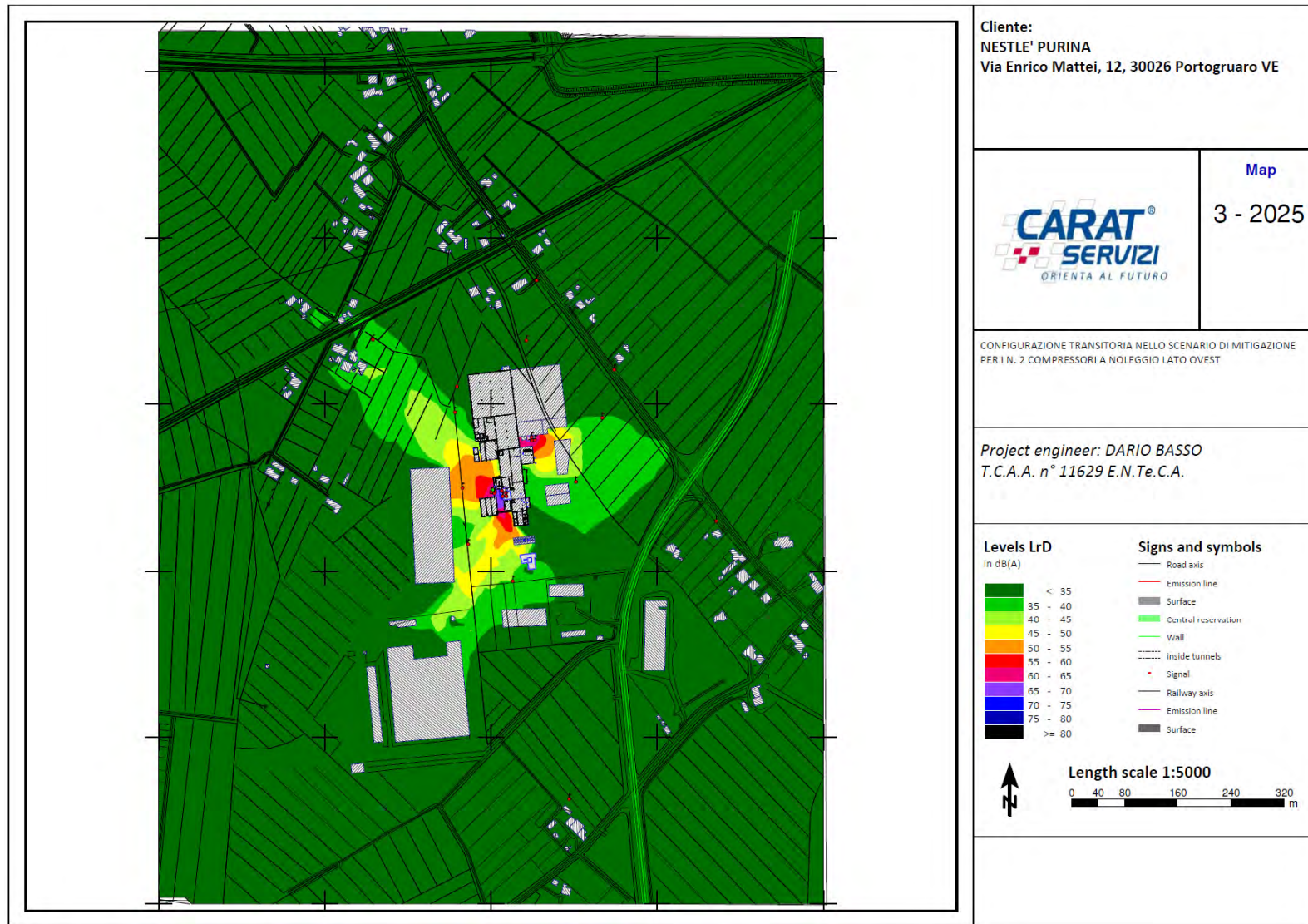
Figura 34 MAPPA IN PIANTA IMPATTO ACUSTICO SCENARIO TRANSITORIO CON INTERVENTO DI MITIGAZIONE – PERIODO DIURNO/NOTTRUNO
