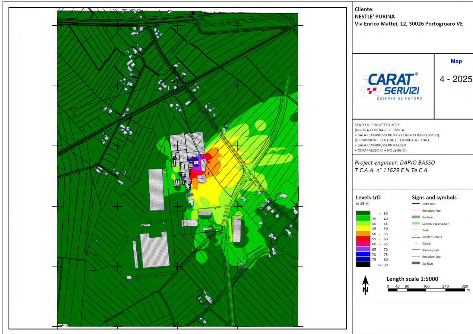
Figura 45 MAPPA IN PIANTA IMPATTO ACUSTICO STATO DI PROGETTO (SORGENTI FISSE: NUOVA CENTRALE TERMICA + SALA COMPRESSORI PKG CON 4 COMPRESSORI E 4 ESTRATTORI D'ARIA) – PERIODO DIURNO / NOTTURNO.
