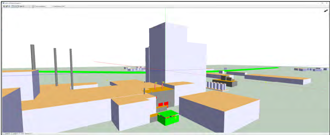
Figura 32 Mappa 3D posizionamento compressori + barriera
