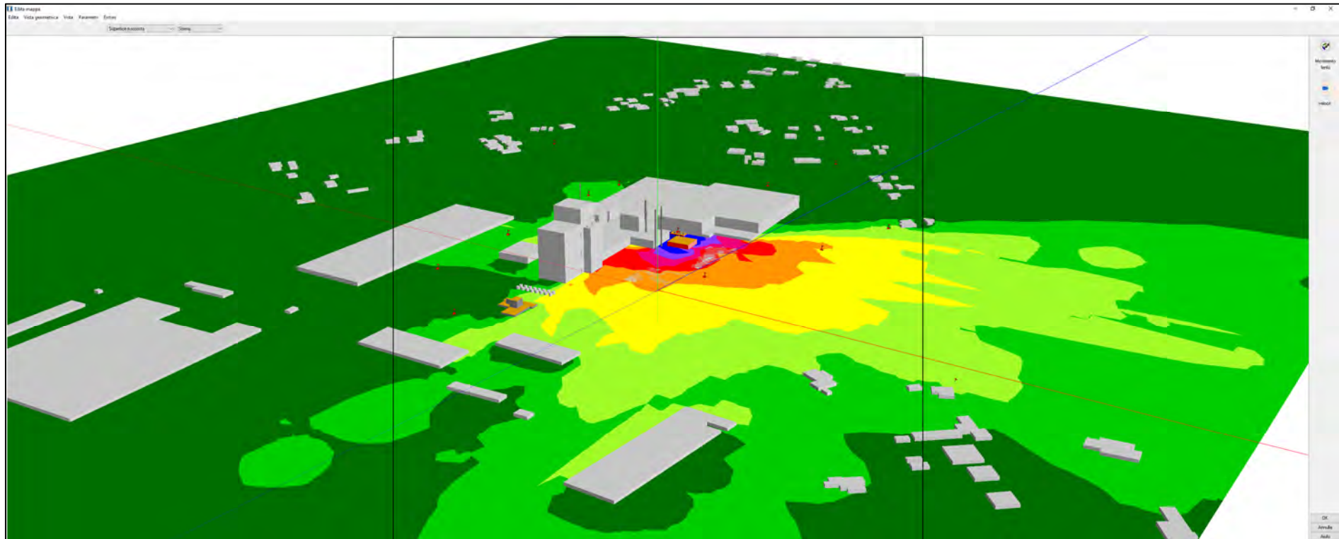
Figura 47 MAPPA 3D IMPATTO ACUSTICO STATO DI PROGETTO (SORGENTI FISSE: NUOVA CENTRALE TERMICA + SALA COMPRESSORI PKG CON 4 COMPRESSORI E 4 ESTRATTORI D'ARIA) – PERIODO DIURNO / NOTTURNO – LATO OVEST
