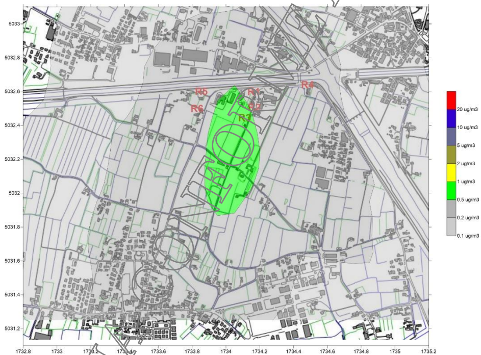
Figura 7 - Risultati della modellizzazione diffusionale. Concentrazione media annua di Acido cloridrico HCl
