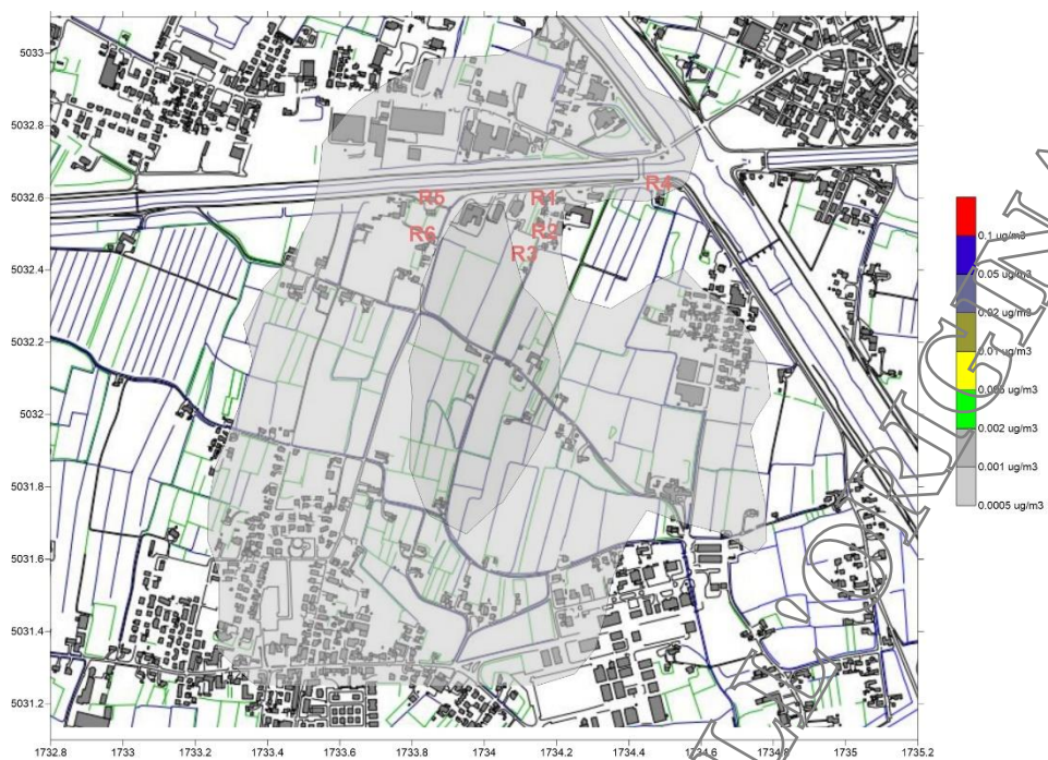
Figura 10 - Risultati della modellizzazione diffusionale. Concentrazione media annua di Cr VI
