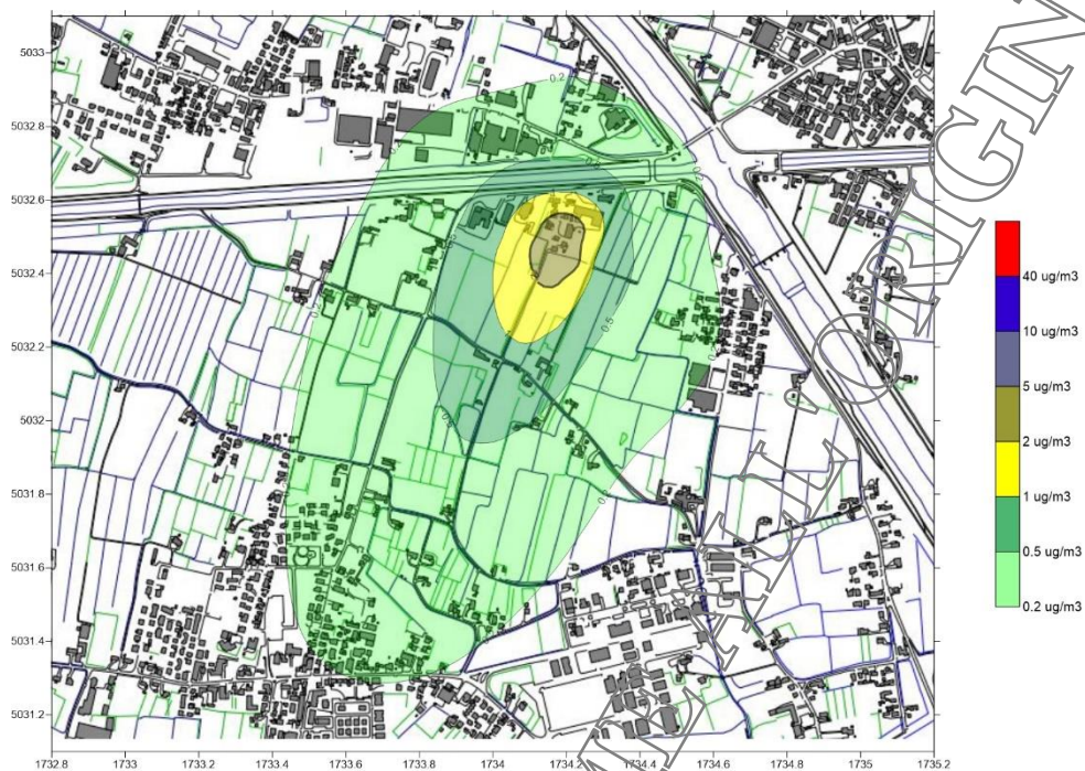
Figura 4 - Risultati della modellizzazione diffusionale. Concentrazione media annua di NO 2 . Scenario cogeneratori A e B
