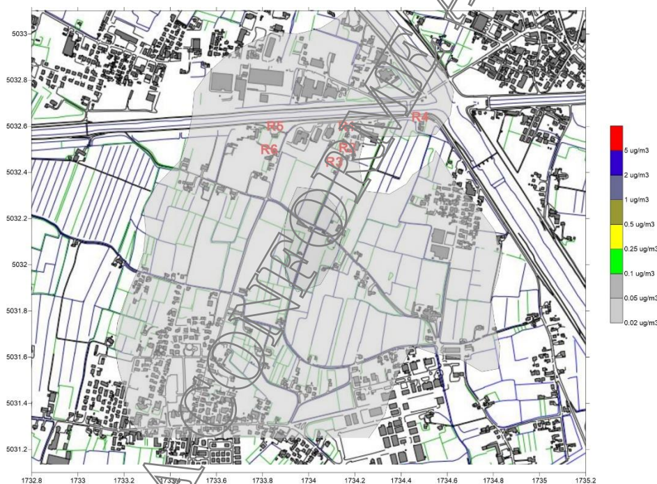
Figura 9 - Risultati della modellizzazione diffusionale. Concentrazione media annua di Cr III
