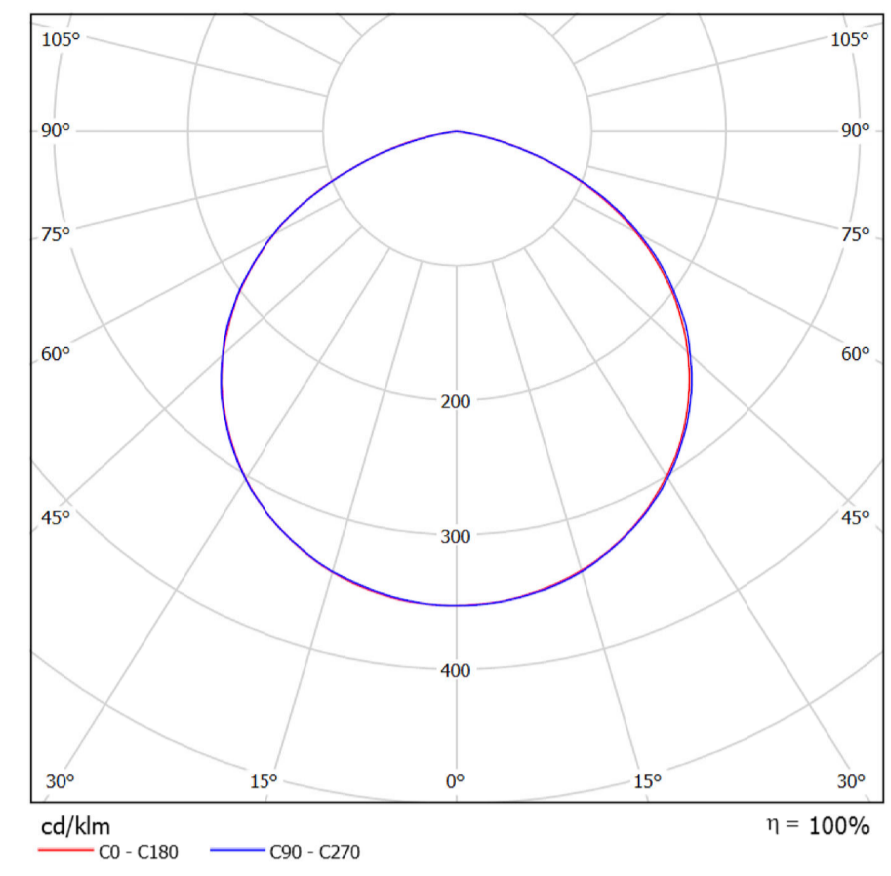
CURVA FOTOMETRICA
